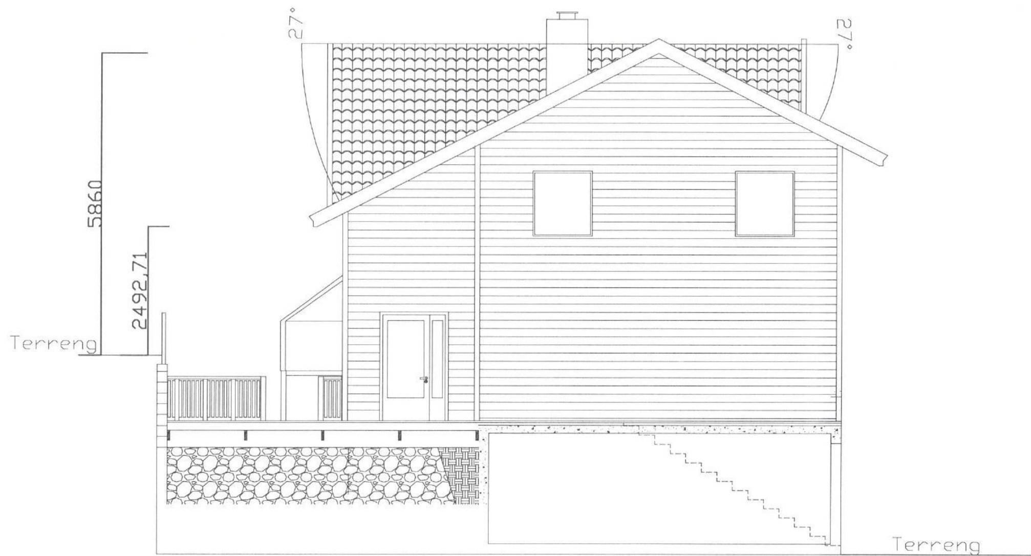
FASEDE NORD ØST
